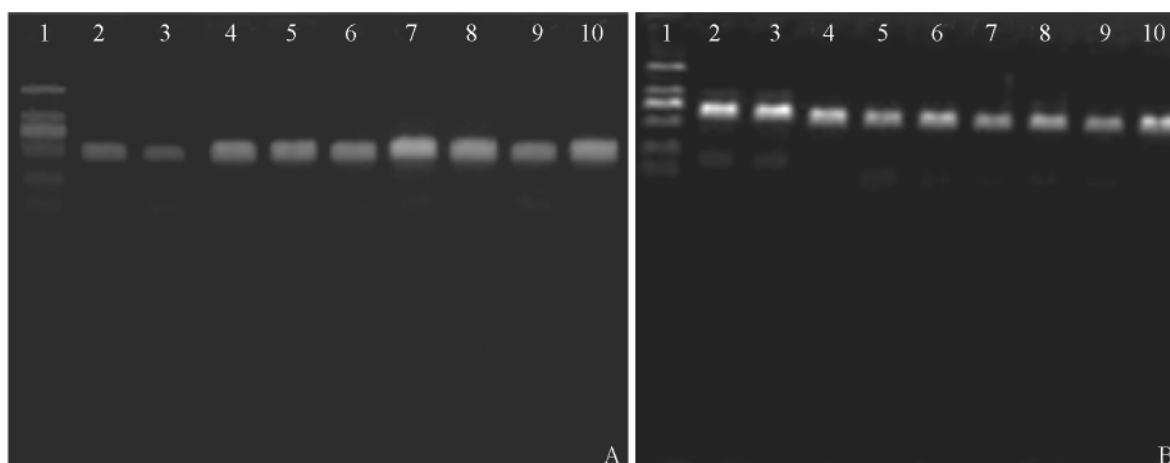
图 2 引物 mtD-7.2F 和 mtD-9.2R 的 STE 法(A)和盐析法(B)扩增结果
