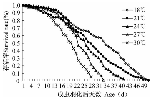
图2 不同温度下绿盲蝽成虫种群存活率曲线
