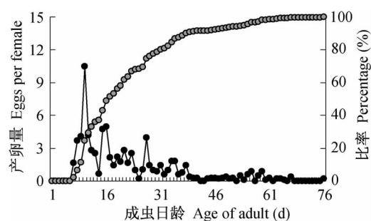
图4 不同日龄绿盲蝽雌性成虫的产卵情况
