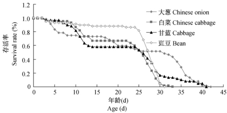
图 1 甜菜夜蛾在不同寄主上的存活率曲线 Fig.1 Survival curves of Spodoptera exigua on different host plants
