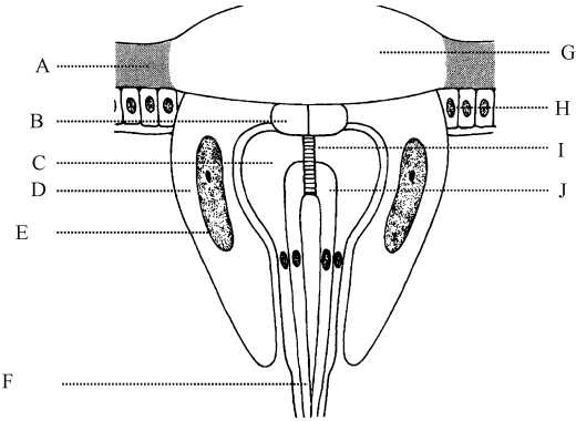
图2 侧单眼的结构示意图(仿 Ro moser)
