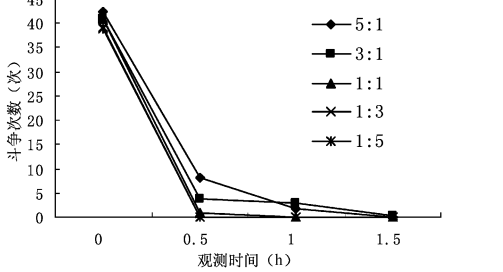
图 1 黑翅土白蚁与台湾乳白蚁工蚁在不同配比下斗争次数随时间的变化
