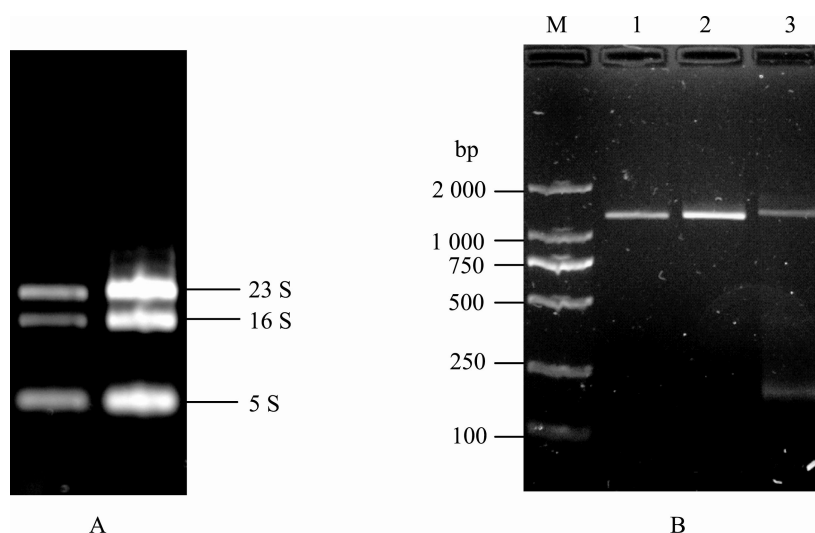
图1 柞蚕微孢子虫 RNA 的提取 (A) 及 \alpha 、 \beta 和 \gamma -微管蛋白基因的 PCR 扩增片段 (B)
