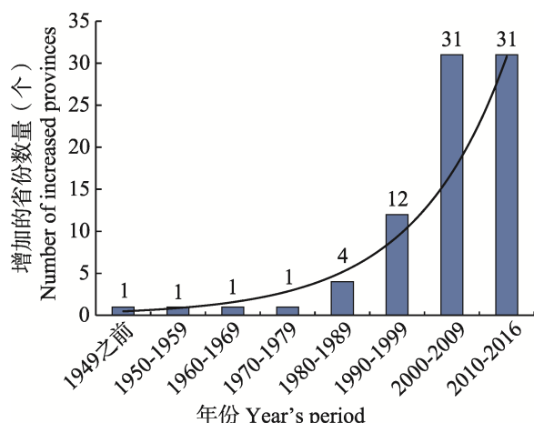
图3 全国农业植物检疫性昆虫传入的省份增长动态
