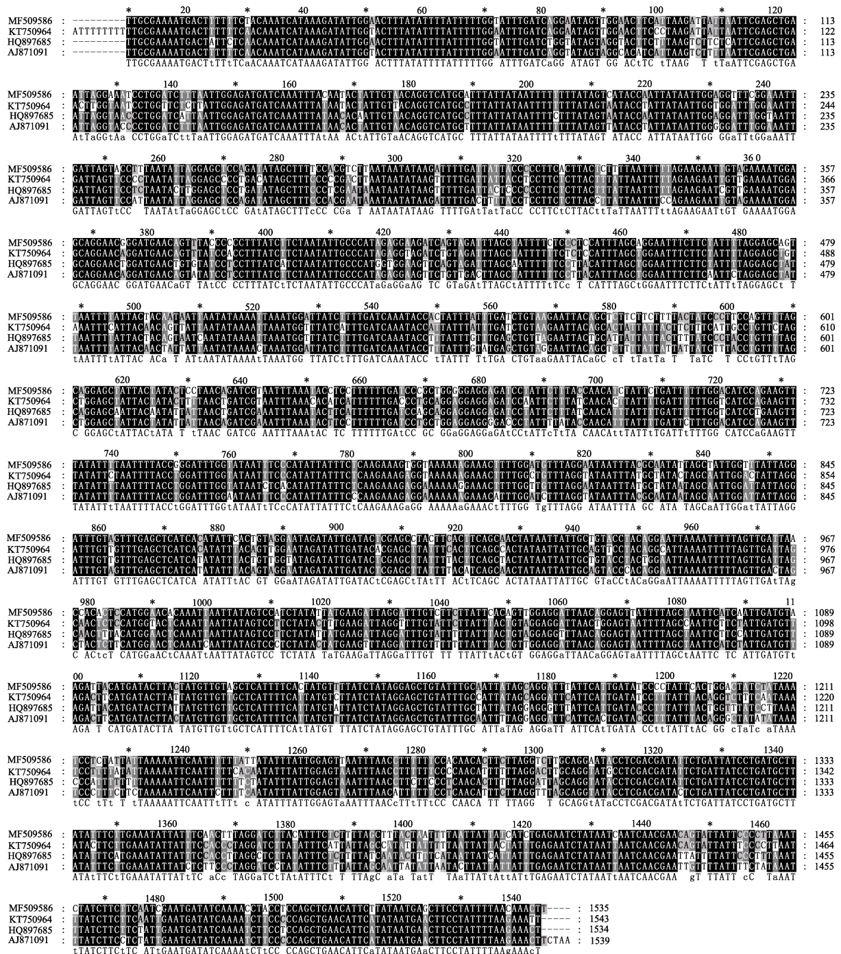
图 2 小蜡螟和其他螟蛾科昆虫 CO I 基因的多序列比对
