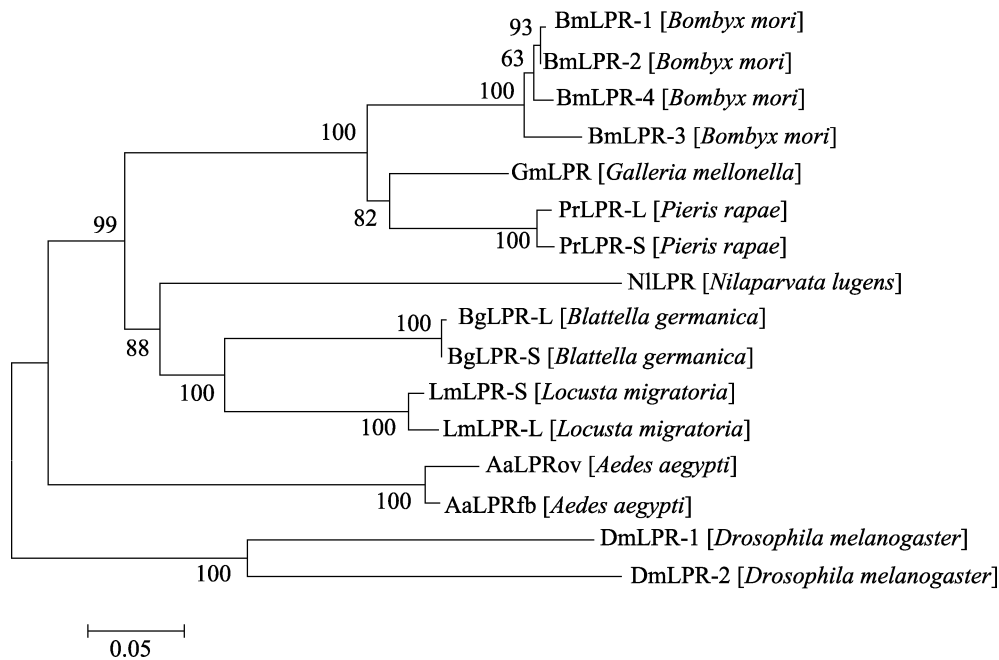
图 3 LmLPR 与其他昆虫载脂蛋白受体 LPR 系统聚类分析
