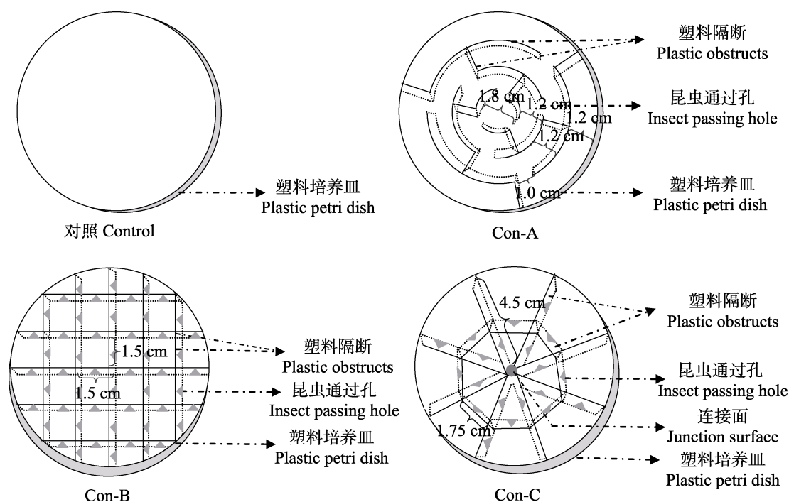
图 1 4 种类型饲养盒的示意图
