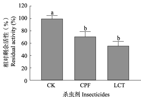
图 4 2 种杀虫剂对 AiGSTs1 重组蛋白活性的抑制效应
