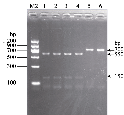
图2 Sap I酶切不同实蝇的mtCO I PCR产物后琼脂糖凝胶电泳图谱
