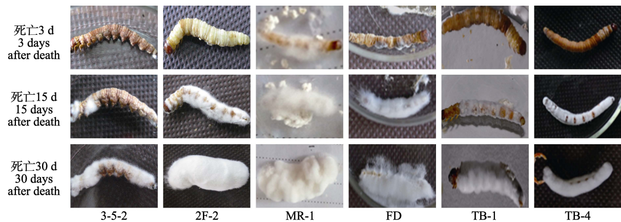
图 4 蝙蝠蛾幼虫被各相关菌感染后的形态
