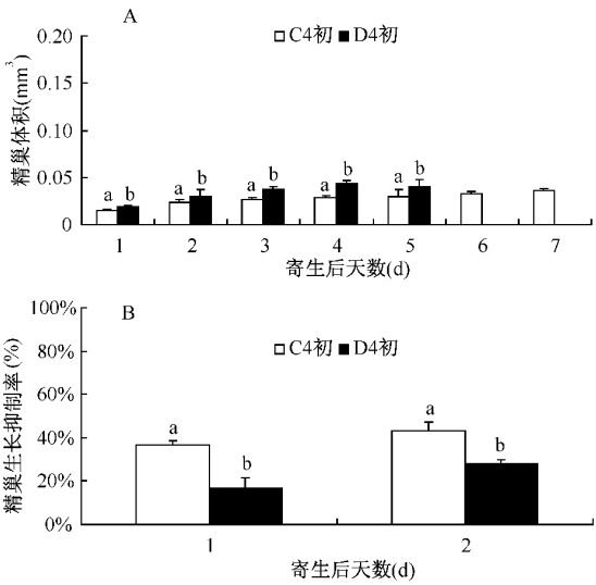
图5 茧蜂和姬蜂寄生4龄初小菜蛾
