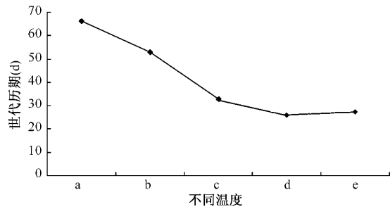
图 1 灰飞虱世代历期与温度关系 a. 15℃ b. 20℃ c. 25℃ d. 28℃ e. 30℃
