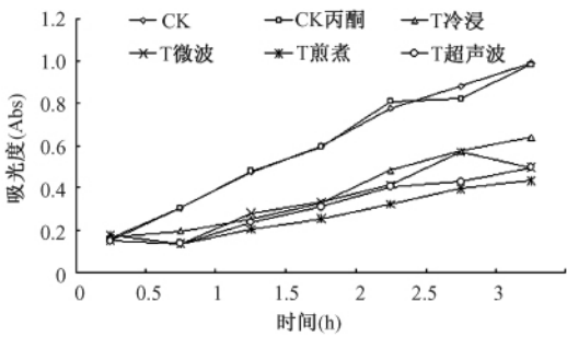
图 1 不同的提取方法得到的蝉蛻提取物活性分析 注:采用 ANOVA 方差分析,显著性差异分析应用 Duncan 多重比较,不同提取方法与对照相比差异显著( P\leq 0.05 ),不同方法之间无显著性差异( P>0.05 )。
