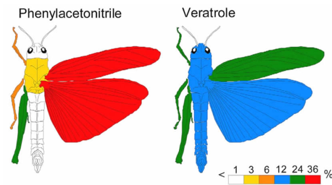
图 2 群居型成熟沙漠蝗雄成虫彩图, 揭示出身体不同部位对苯乙腈 (phenylacetonitrile) 和藜芦醚 (veratrole) 总释放量的相对贡献 (Seidelmann et al. , 2003)
