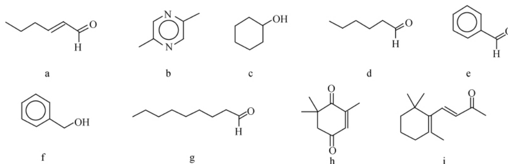
图 3 已报道的东亚飞蝗虫粪挥发物电生理活性组分
