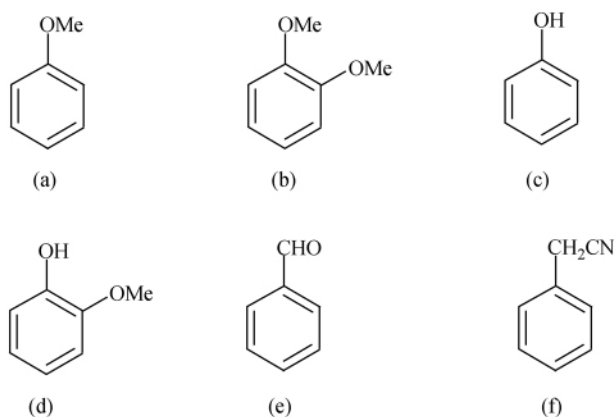
图 1 群集型沙漠蝗成虫体挥发物组分
