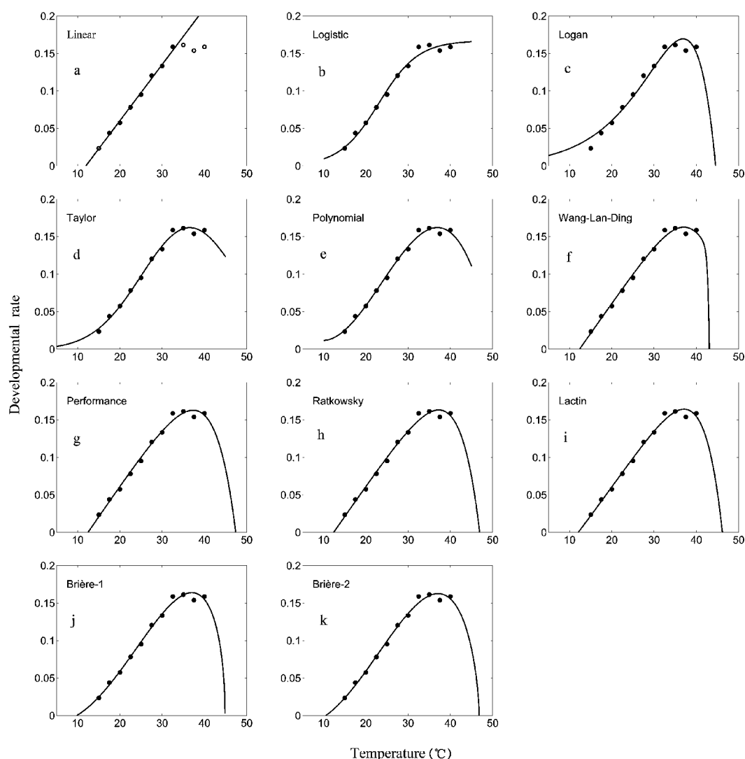
图 1 不同数学模型对发育速率数据的拟合
