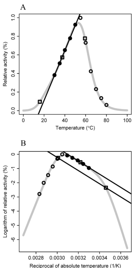
图4 SSI模型对不同温度下棕榈象甲 Rhynchophorus palmarum 消化液中的 \beta -半乳糖苷酶类活性影响的描述(Yapi et al. , 2007)
