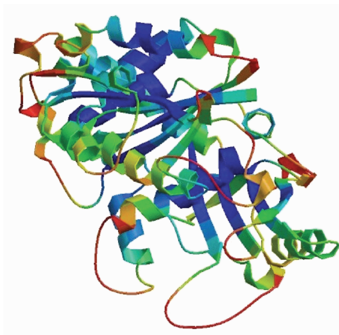
图 2 棉铃虫 \beta -微管蛋白三维结构带状图
