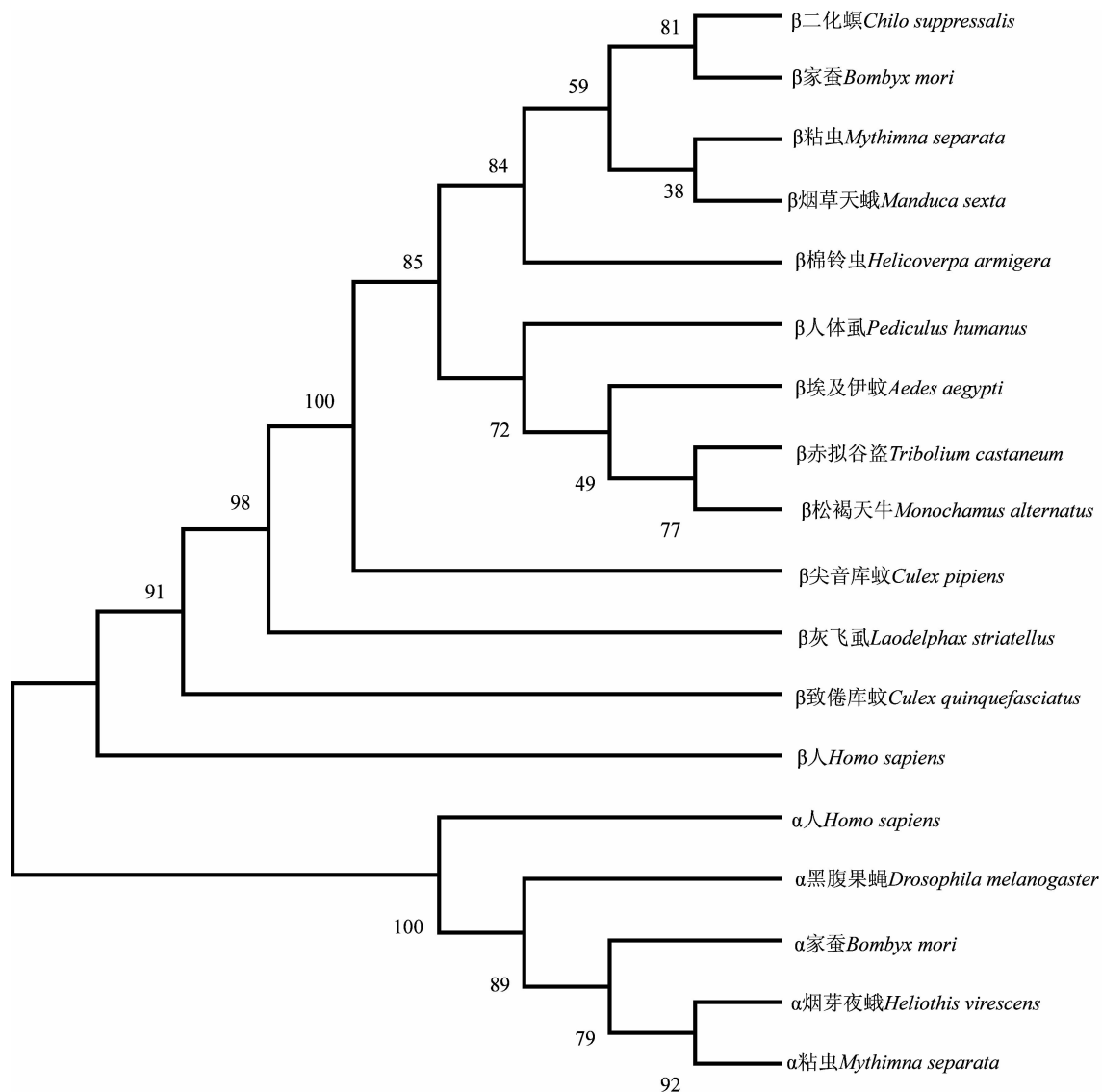
图3 基于 \alpha 、 \beta -微管蛋白氨基酸序列的 Neighbor-Joining 系统树(分支点数值为置信度值)
