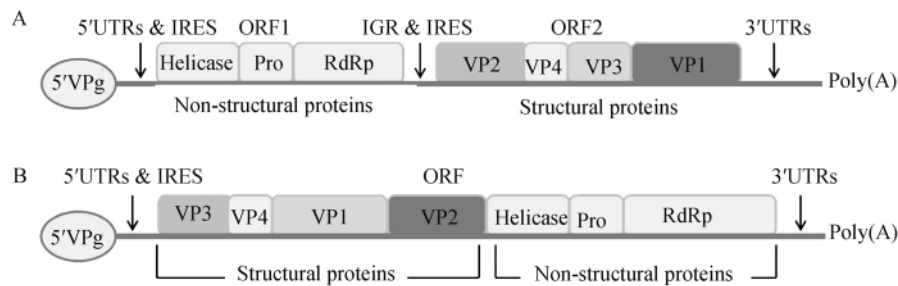
图 2 2 种蜜蜂病毒属的基因组结构与功能示意图
