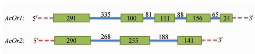
图 1 AcOr1 和 AcOr2 的基因结构模式图
