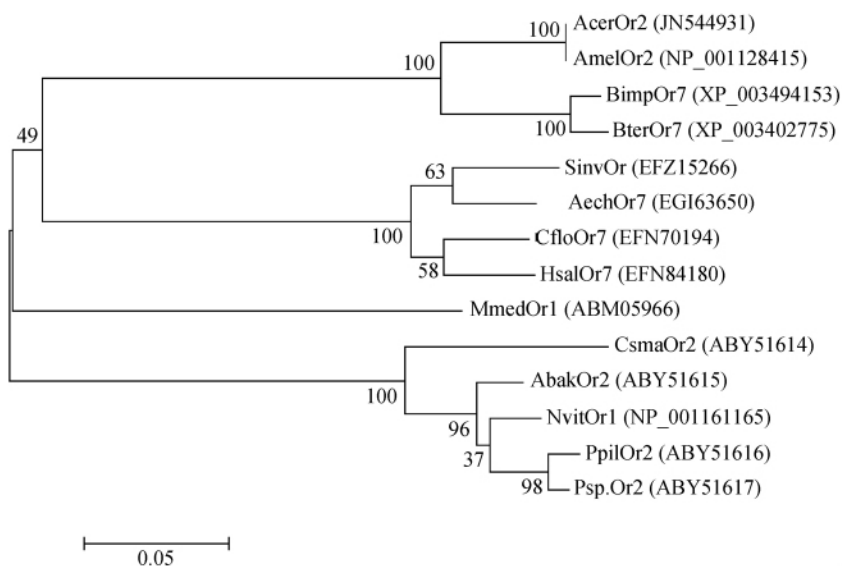
图 7 AcOr2 与其同源序列的系统进化树
