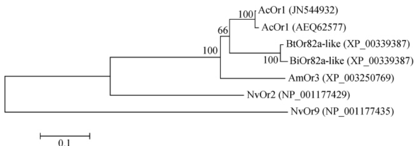
图 6 AcOr1 与其同源序列的系统进化树
