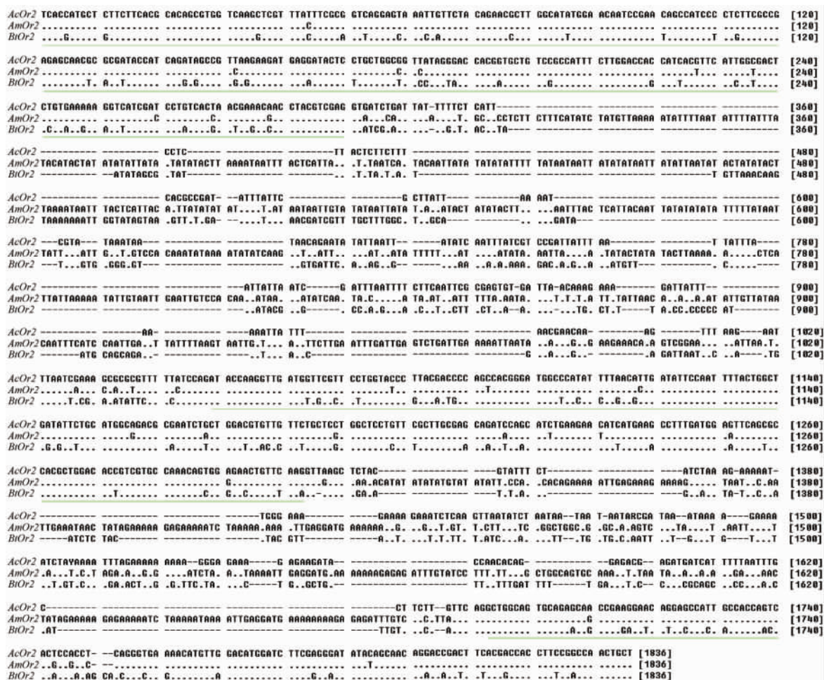
图3 AcOr2 核苷酸序列与其它昆虫相应序列的比对
