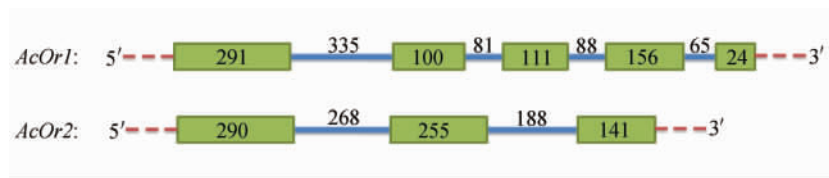
图 1 AcOr1 和 AcOr2 的基因结构模式图
