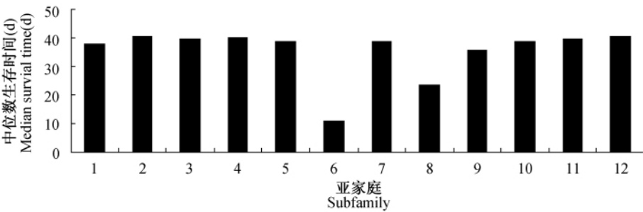
图 1 亚家庭中位生存时间 Fig.1 Median survival time of subfamilies
