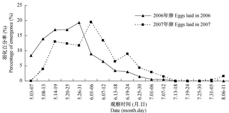
图2 松褐天牛成虫在第2年的羽化规律
