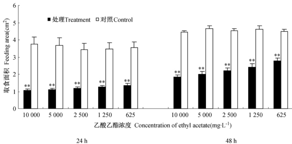
图 1 乙酸乙酯提取物对小菜蛾 3 龄幼虫在甘蓝植株上的拒食活性(选择性试验)
