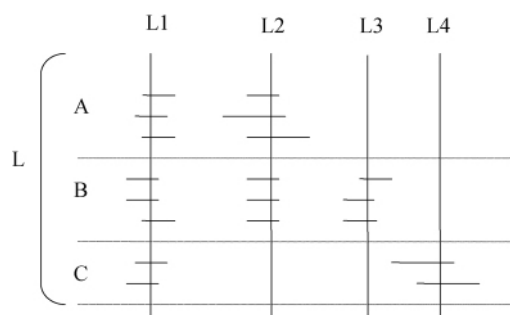
图 2 4 类 L-fibers 在神经节各亚层内的分支 Fig. 2 Lateral processes of four types of L-fibers in different lamina strata
