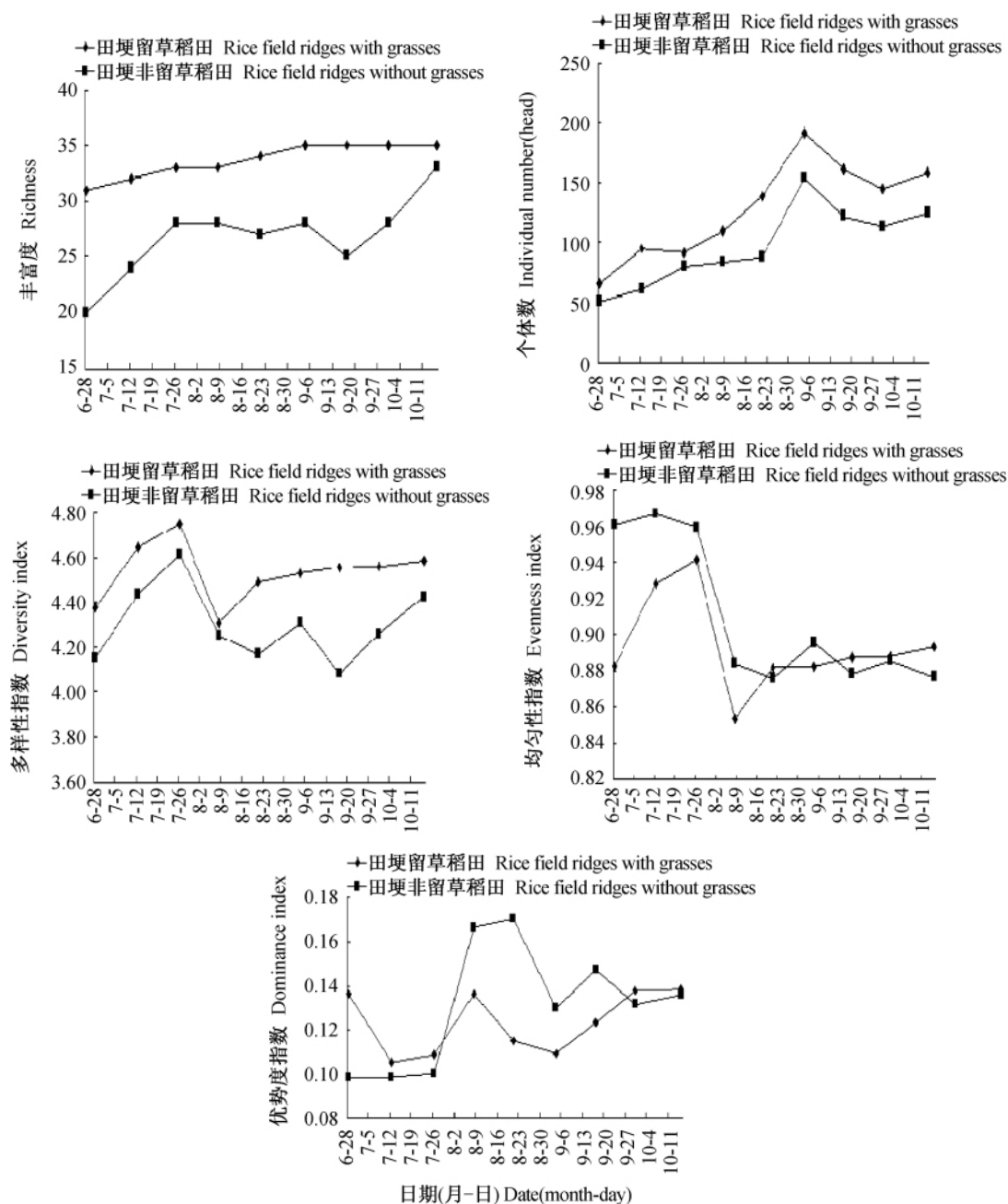
图3 不同类型稻田捕食性天敌结构特征值动态变化
