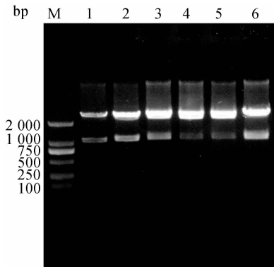
图 2 东亚飞蝗 AK 克隆载体经 EcoR I 和 Xho I 双酶切鉴定 Fig.2 Restriction analysis for pMD18-T-AK with EcoR I and Xho I of Locusta migratoria manilensis M: DNA (DL2000) 标志物;1~6:克隆载体经 EcoR I 和 Xho I 双酶切后。 M: DNA marker (DL2000); 1-6: pMD18-T-AK/ EcoR I + Xho I.
