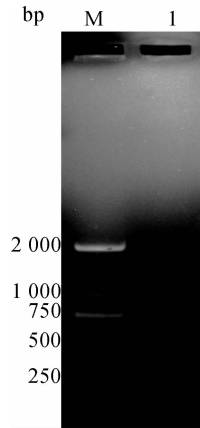
图 1 东亚飞蝗 AK 的 RT-PCR 产物电泳图 Fig.1 RT-PCR products of arginine kinase (AK) of Locusta migratoria manilensis M: DNA (DL2000) 标志物;1: 目的基因。 M: DNA marker (DL2000); 1: target genes.
