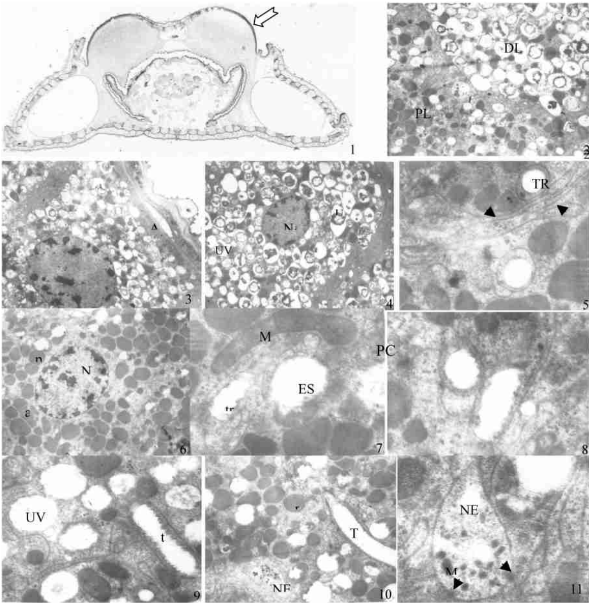
图版Ⅲ 条背萤幼虫发光器结构
