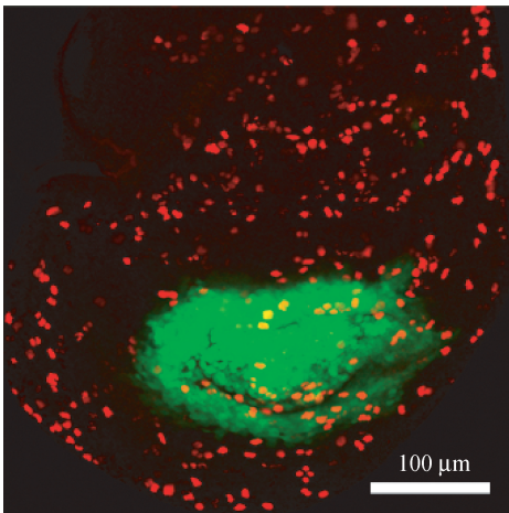
图 7 共表达 GFP(绿)、P35 和 brinker 基因的翅芽的 PH3 染色(红)
