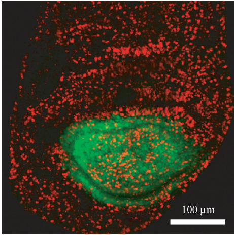
图 6 共表达 GFP(绿)、P35 和 brinker 基因的翅芽的 BrdU 染色(红)
