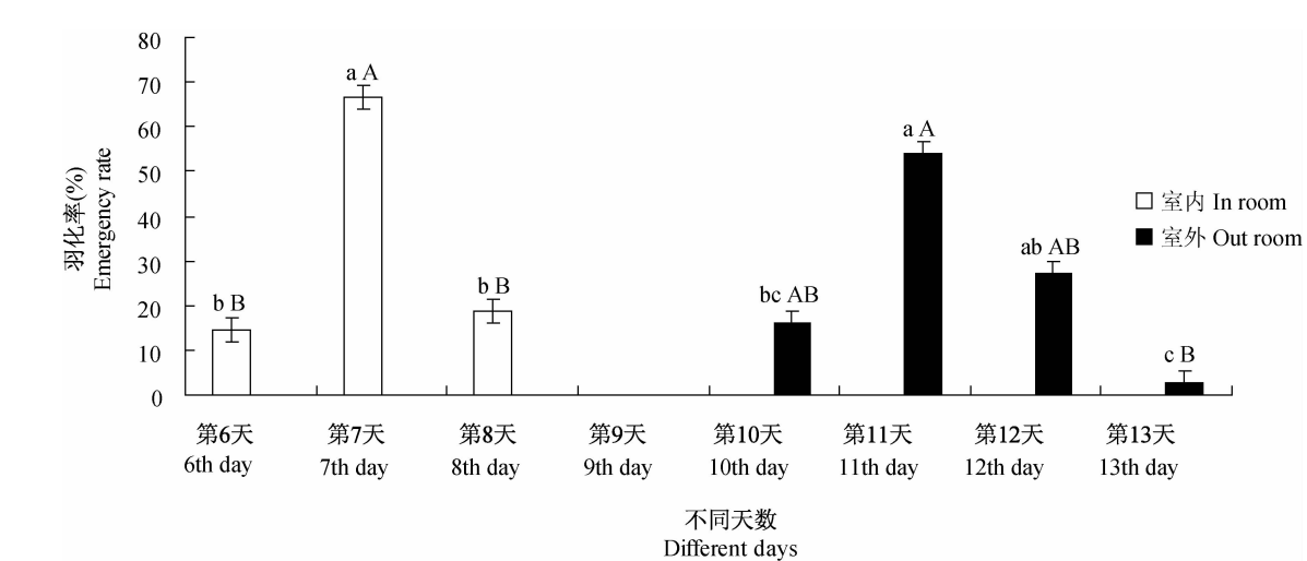
图 4 梨小食心虫在室内和室外条件下不同天数羽化率比较
