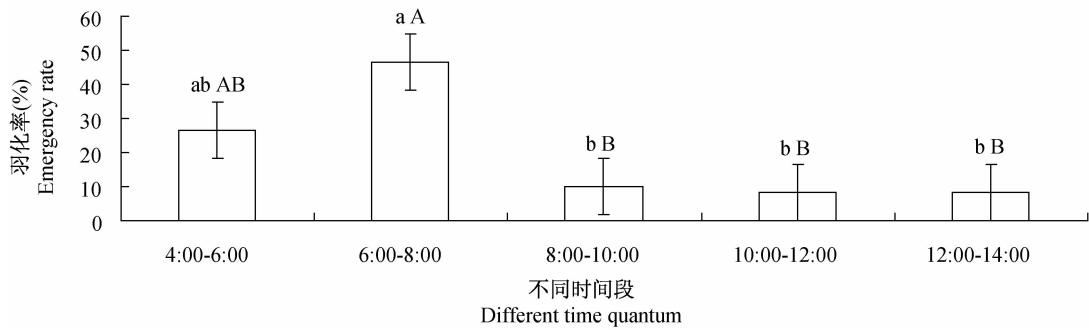
图 2 桃园采集梨小食心虫不同时间段羽化率
