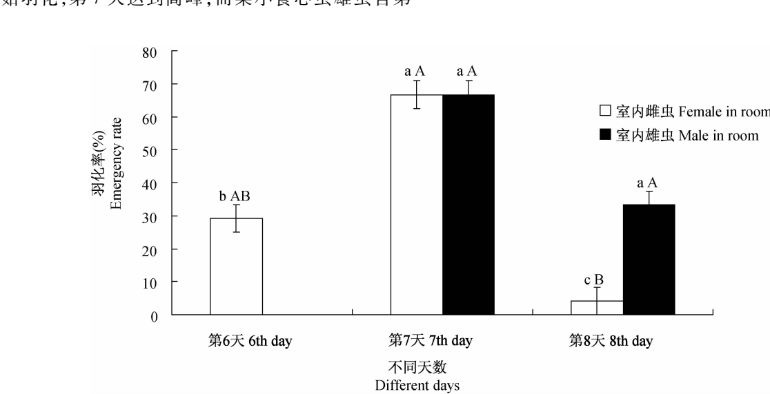
图 5 室内饲养梨小食心虫不同天数羽化雌雄比
