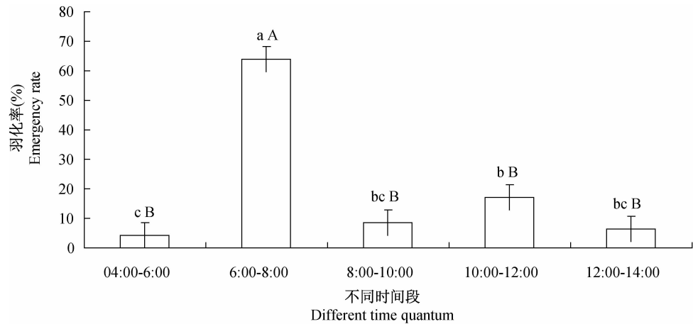
图 1 室内饲养梨小食心虫不同时间段羽化率
