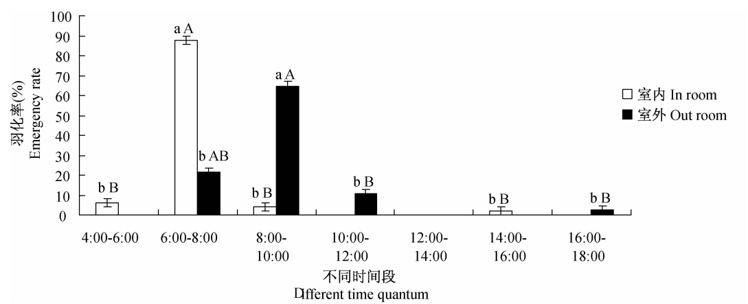
图 3 梨小食心虫在室内和室外条件下不同时间段羽化率比较
