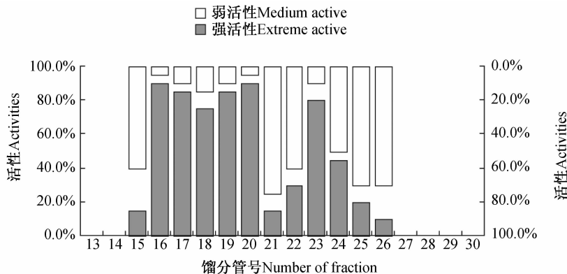
图 2 硅胶柱层析分离馏分的生物活性测定结果
