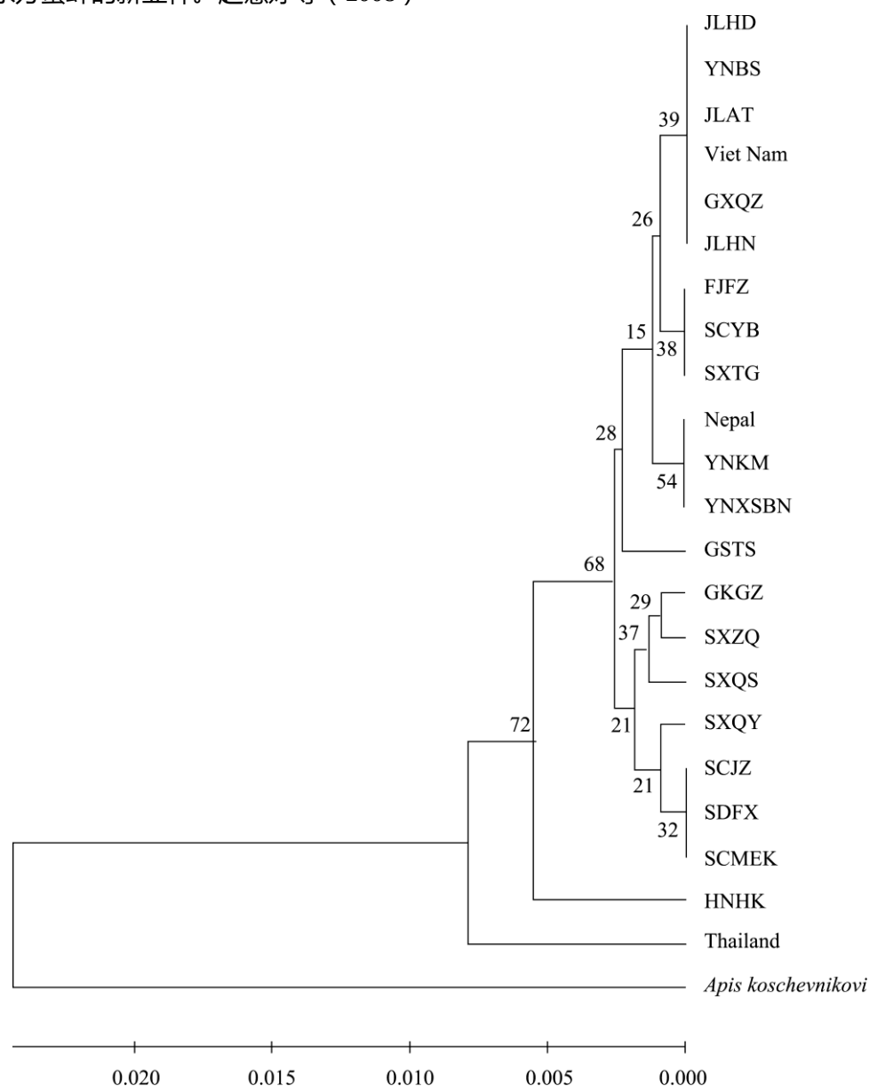
图 6 基于 tRNA^{Ile}\sim ND_2 部分基因序列以 UPGMA 法所构建的系统发育树
