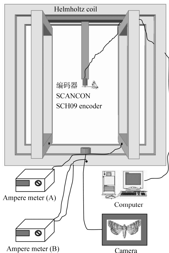
图 1 定向试验装置包括亥姆霍兹线圈、编码器、红外摄像头和悬吊装置 4 个主要部分
