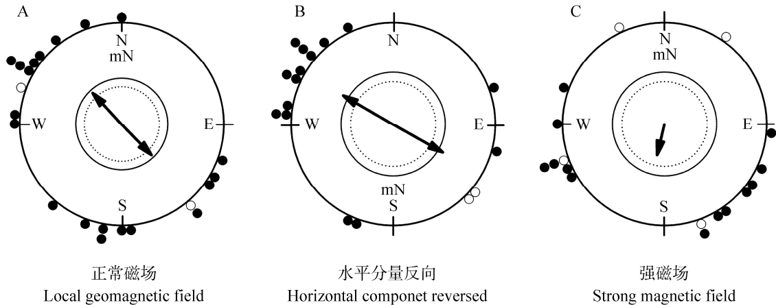
图 2 公主岭粘虫自然种群在不同磁场中的定向行为
