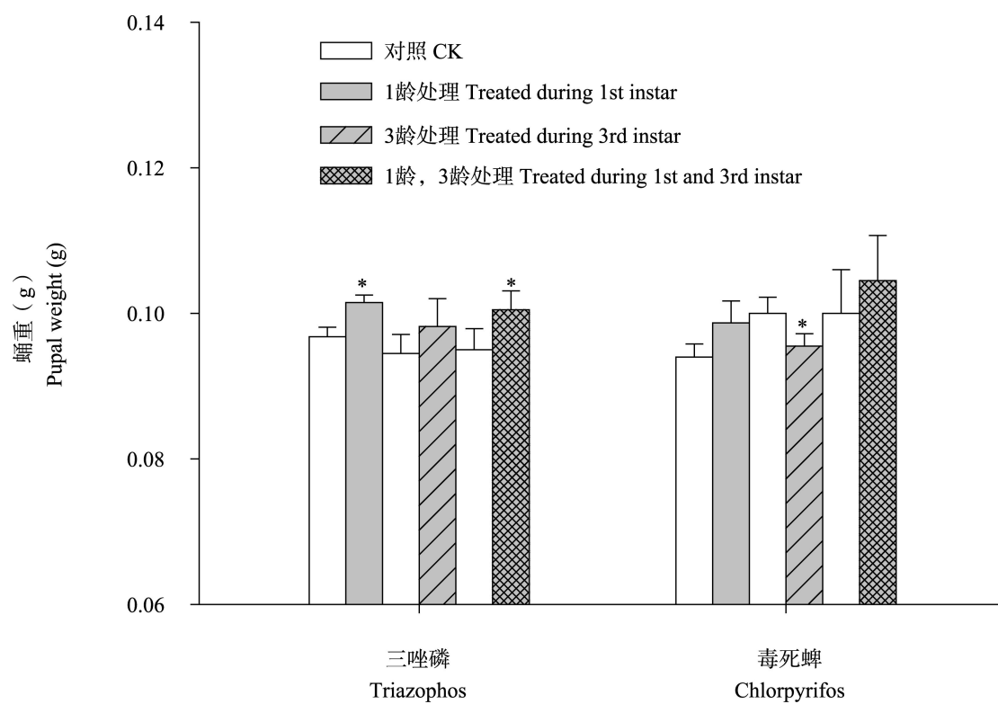
图 2 三唑磷和毒死蜱处理对大螟蛹重的影响
