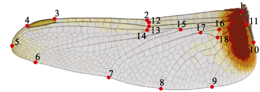
图 2 黄蜻后翅形态测量的地标志点 Fig. 2 Distribution of landmarks on hindwing of Pantala flavescens
