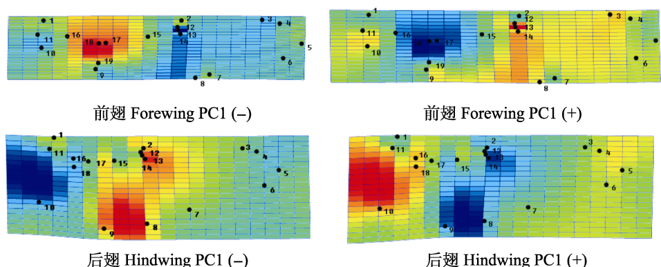
图5 黄蜻雌雄性前后翅的 TPS 分析
