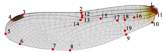
图 1 黄蜻前翅形态测量的地标志点 Fig. 1 Distribution of landmarks on forewing of Pantala flavescens
