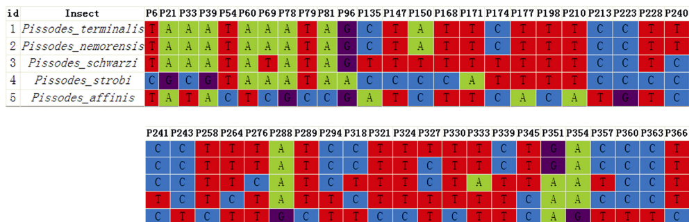
图 3 木蠹象属昆虫的鉴定特征 (CO 基因片段长度 371 bp)
