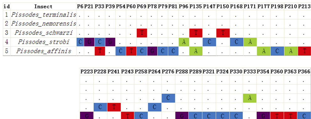
图 4 木蠹象属昆虫的标记性碱基信息 (CO 基因片段长度 371 bp)
