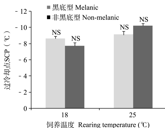
图1 两种发育温度( 18^{\circ}\text{C} 和 25^{\circ}\text{C} )下不同色斑型成虫的过冷却点
