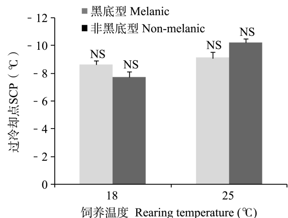
图1 两种发育温度(18℃和25℃)下不同色斑型成虫的过冷却点
