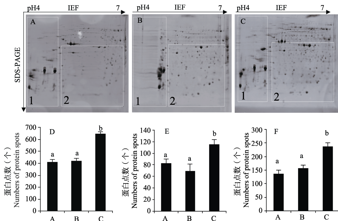
图 1 TCA-丙酮 3 种蛋白提取方法的 2-DE 图谱比较
