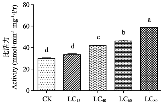
图4 乙基多杀菌素对棉铃虫乙酰胆碱酯酶 (AChE) 酶比活力的影响
