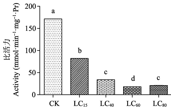
图 1 乙基多杀菌素对棉铃虫羧酸酯酶 (CarE) 比活力的影响
