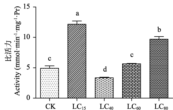
图 3 乙基多杀菌素对棉铃虫多功能氧化酶 (MFO) 酶比活力的影响
