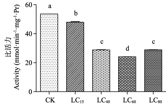
图 2 乙基多杀菌素对棉铃虫谷胱甘肽-S-转移酶 (GST) 比活力的影响
