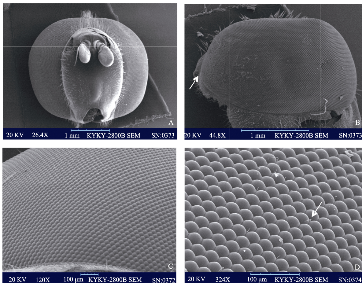
图 2 黑带食蚜蝇复眼扫描电镜照片
