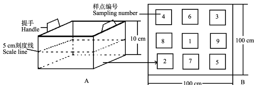
图 3 底栖昆虫采样方法示意图
