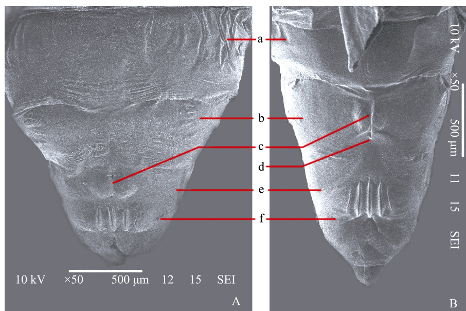
图 2 扫描电镜观察的雌雄蛹腹部末端（腹面观）
