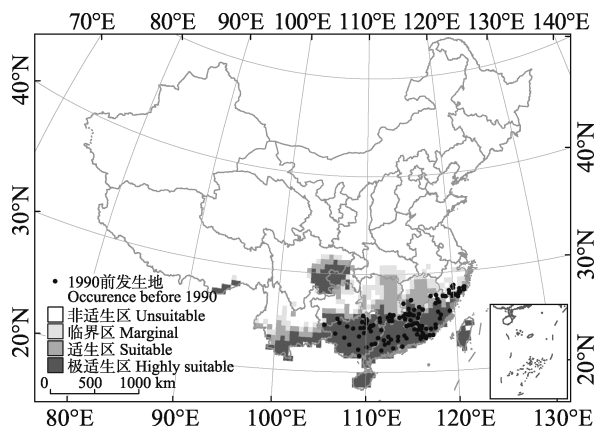
图4 1990年 CLIMEX 模拟柑橘木虱适生区与实际发生地
