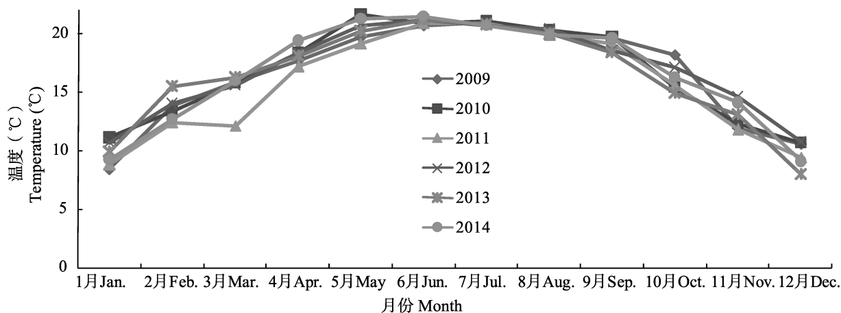
图4 2009—2014年通海县月平均气温曲线
