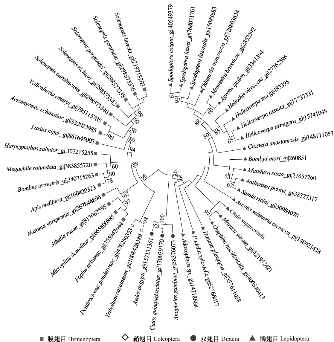
图 2 昆虫 PBAN 前体肽序列的系统进化树构建
