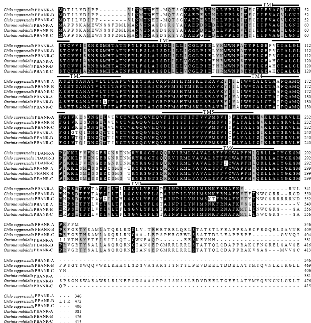
图 4 二化螟和玉米螟 PBAN 受体氨基酸序列比对
