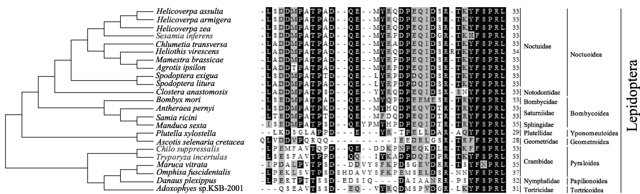
图 3 鳞翅目昆虫 PBAN 成熟肽序列比对和进化树分析
