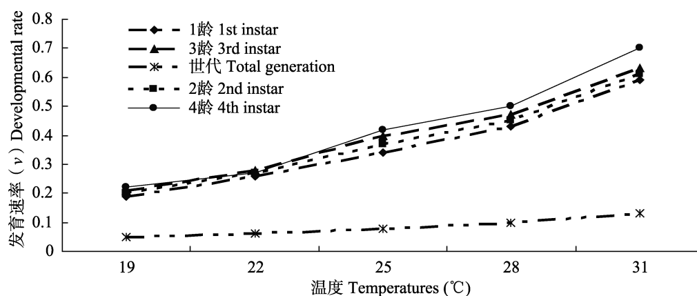
图1 不同温度下胡萝卜微管蚜发育速率比较(2015, 沈阳)
