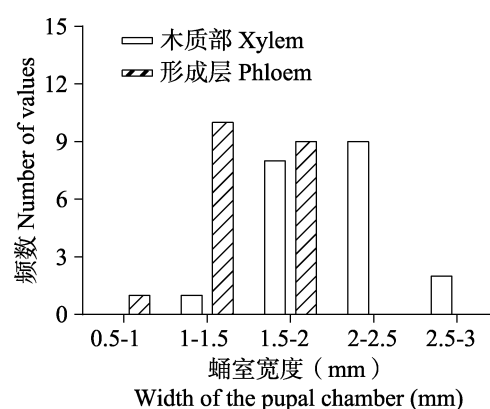
图 6 位于木质部和韧皮部蛹室宽度的频次分布图
