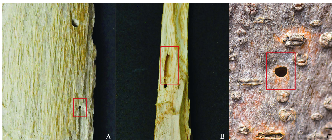
图 7 示合欢吉丁的侵入孔、蛹室和羽化孔
